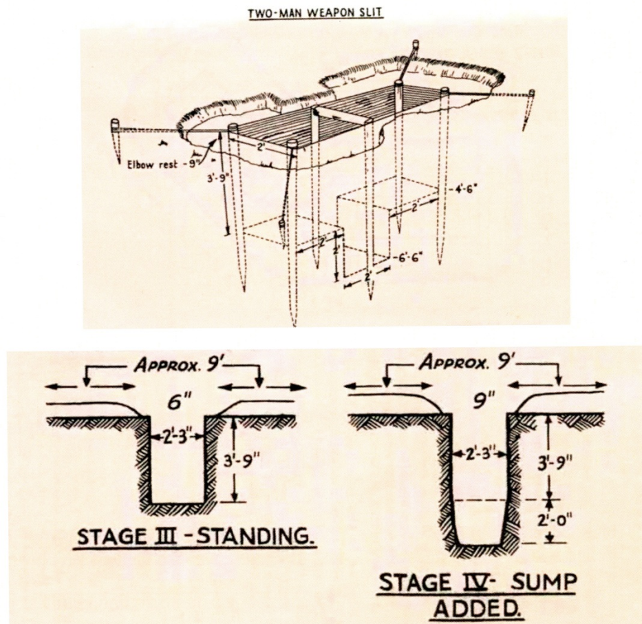
Afb. 5.7 en 5.8. Fragmenten uit een Brits voorschrift met daarop twee voorbeelden van een zogeheten "weapon slit", in feet en inches (bron: The War Office 1944).
