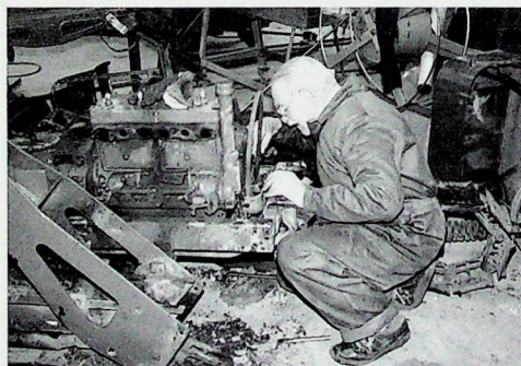
Jaap Jansen bezig met het demonteren van de motor van de Clarkair bulldozer.
